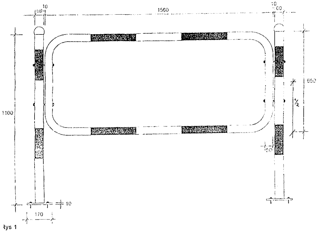
Rys. 1 Poręcz ochronna sztywne z pochwytem i przeciągiem
