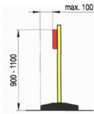
Rys. 6. Ustawienie zapory drogowej U-20
