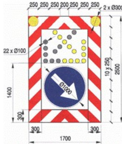
Rys. 16. Wzór tablicy zamykającej U-26b Rys. 17. Tablica zamykająca U-26c
