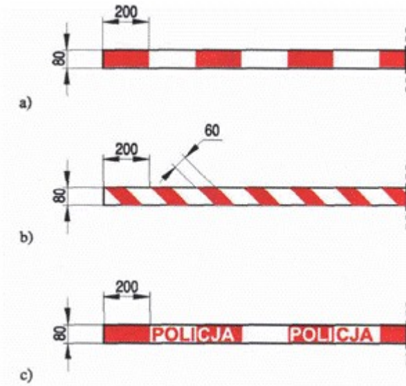
Rys. 8. Przykłady taśm ostrzegawczych U-22
