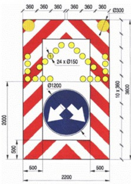
Rys. 16. Wzór tablicy zamykającej U-26b Rys. 17. Tablica zamykająca U-26c
