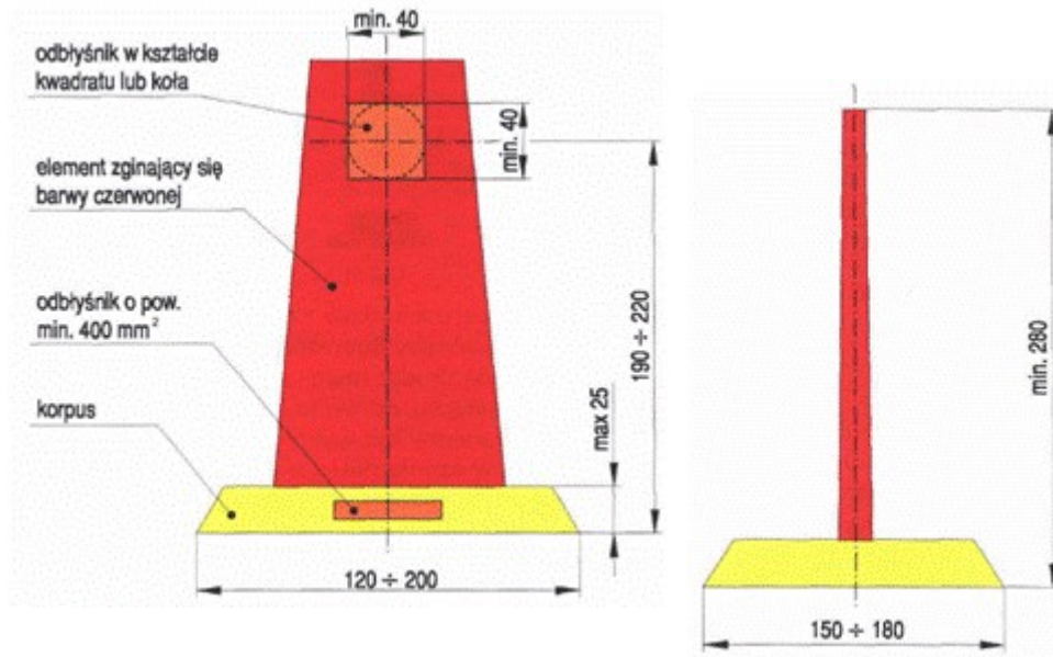
Rys. 11. Tablica uchylna z elementami odblaskowymi U-24
